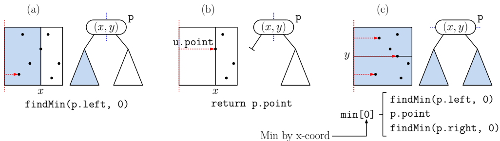
Fig. 75: Cases in findMin .
