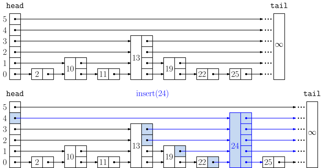
Fig. 61: Inserting a new key 24.
